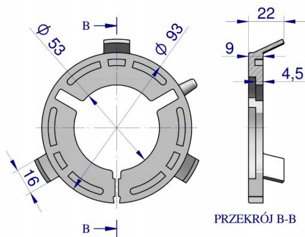
Pierścień wewnętrzny
