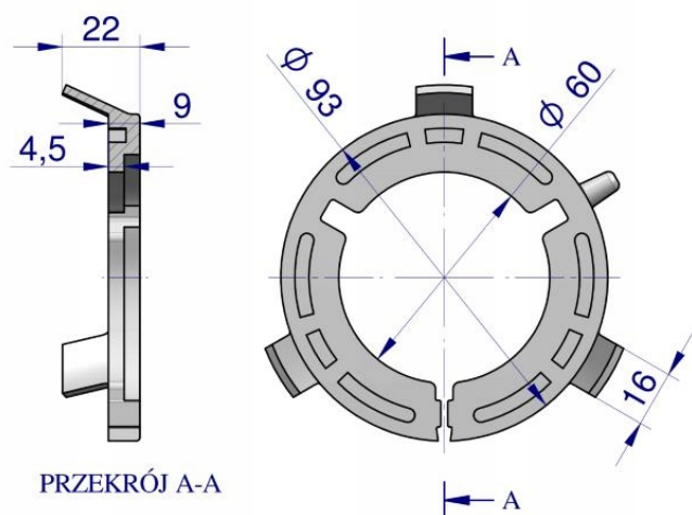
Pierścień zewnętrzny
