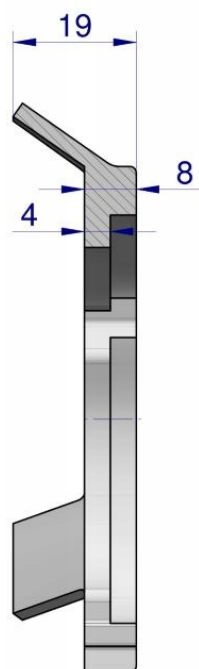
PRZEKRÓJ A-A
