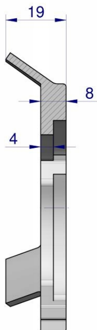
PRZEKRÓJ A-A
