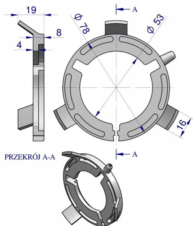
Pierścień zewnętrzny
