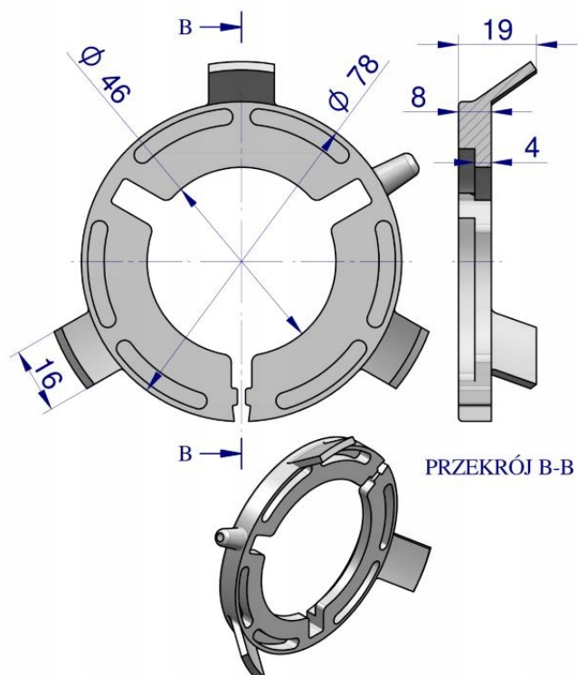
Pierścień wewnętrzny
