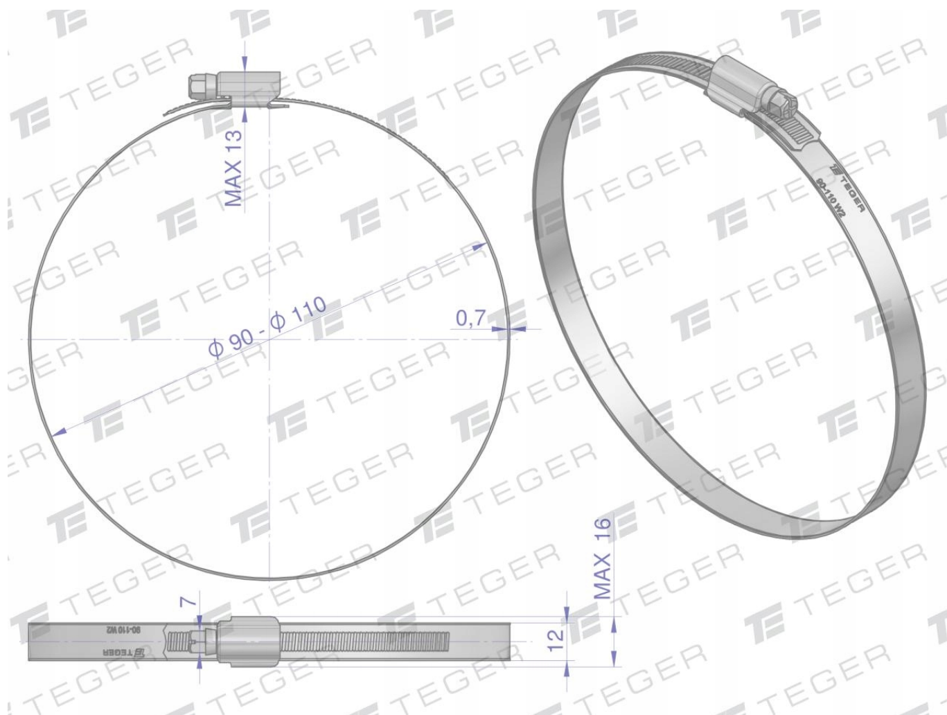
Opaska zaciskowa wzmacniana 90-110 ślimakowa skręcana (obejma W2 - stal nierdzewna) szerokość 12mm TEGER. Opaski zaciskowe ślimakowe - łatwe w montażu: śrubokręt lub klucz, trwałe, duża siła zaciskająca.
