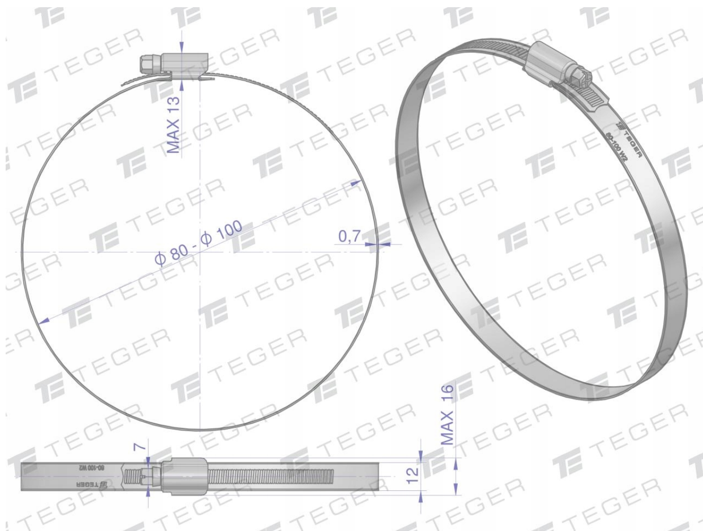
Opaska zaciskowa wzmacniana 80-100 ślimakowa skręcana (obejma W2 - stal nierdzewna) szerokość 12mm TEGER. Opaski zaciskowe ślimakowe - łatwe w montażu: śrubokręt lub klucz, trwałe, duża siła zaciskająca.
