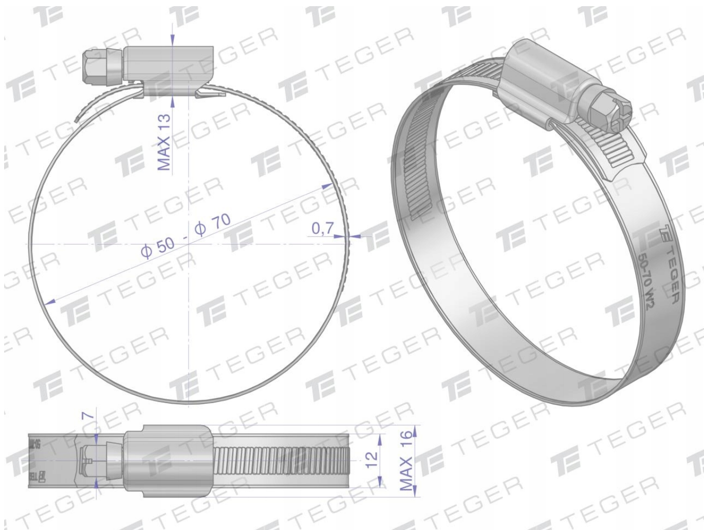
Opaska zaciskowa wzmacniana 50-70 ślimakowa skręcana (obejma W2 - stal nierdzewna) szerkość 12mm TEGER. Opaski zaciskowe ślimakowe - łatwe w montażu: śrubokręt lub klucz, trwałe, duża siła zaciskająca.
