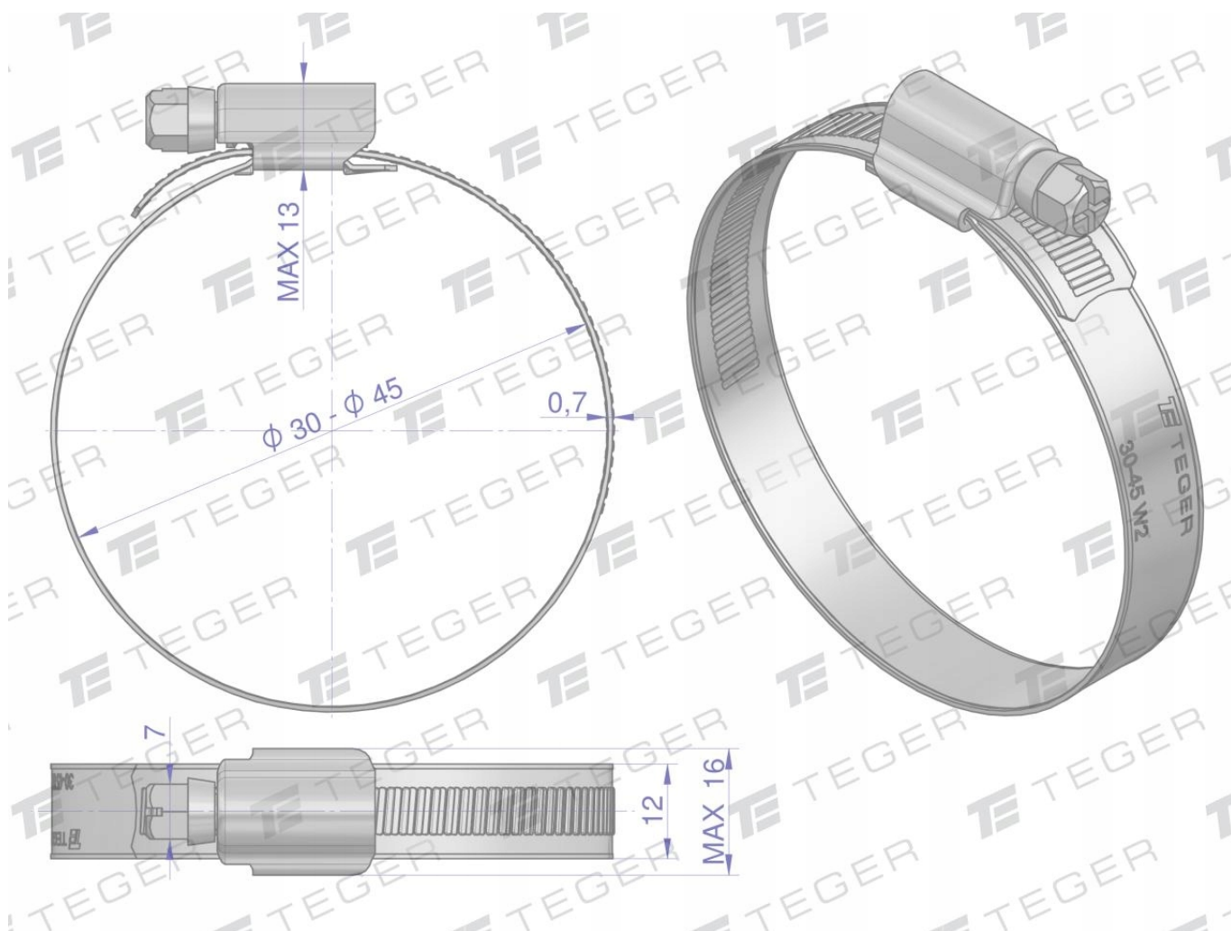
Opaska zaciskowa wzmacniana 30-45 ślimakowa skręcana (obejma W2 - stal nierdzewna) szerkość 12mm TEGER. Opaski zaciskowe ślimakowe - łatwe w montażu: śrubokręt lub klucz, trwałe, duża siła zaciskająca.
