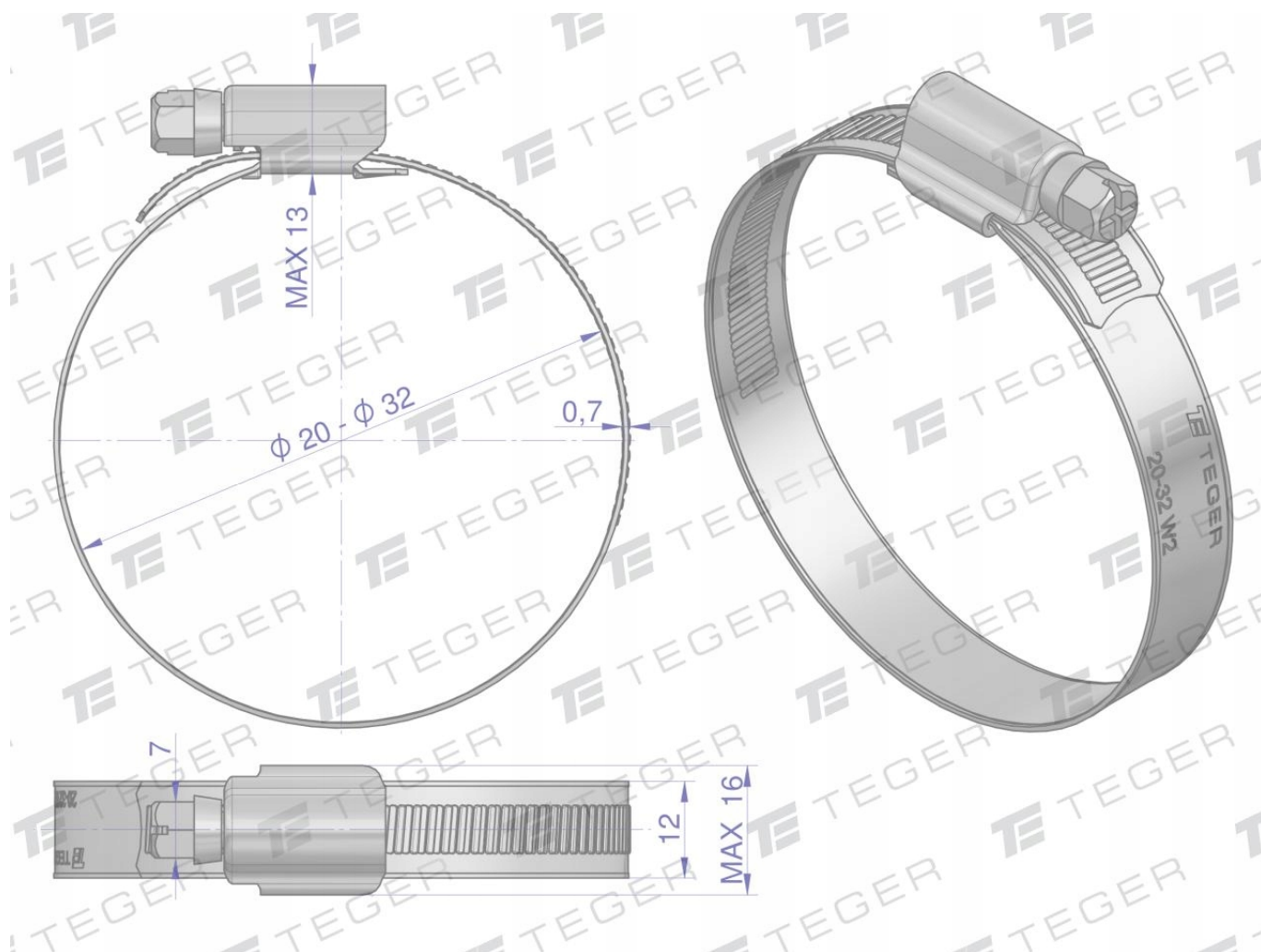
Opaska zaciskowa wzmacniana 20-32 ślimakowa skręcana (obejma W2 - stal nierdzewna) szerkość 12mm TEGER. Opaski zaciskowe ślimakowe - łatwe w montażu: śrubokręt lub klucz, trwałe, duża siła zaciskająca.
