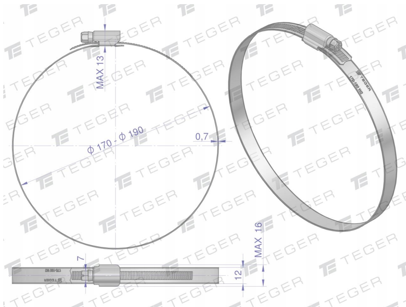
Opaska zaciskowa wzmacniana 170-190 ślimakowa skręcana (obejma W2 - stal nierdzewna) szerkość 12mm TEGER. Opaski zaciskowe ślimakowe - łatwe w montażu: śrubokręt lub kluczyk, trwałe, duża siła zaciskająca.
