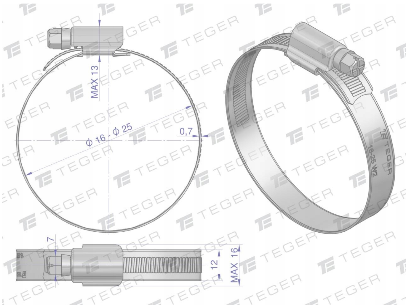
Opaska zaciskowa wzmacniana 16-25 ślimakowa skręcana (obejma W2 - stal nierdzewna) szerkość 12mm TEGER. Opaski zaciskowe ślimakowe - łatwe w montażu: śrubokręt lub klucz, trwałe, duża siła zaciskająca.
