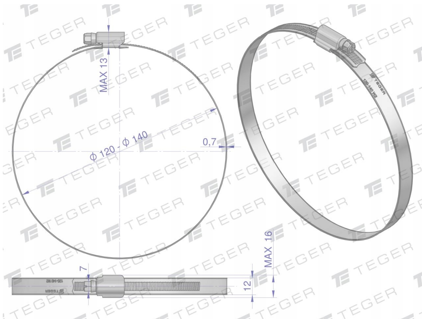
Opaska zaciskowa wzmacniana 120-140 ślimakowa skręcana (obejma W2 - stal nierdzewna) szerkość 12mm TEGER. Opaski zaciskowe ślimakowe - łatwe w montażu: śrubokręt lub kluczyk, trwałe, duża siła zaciskająca.
