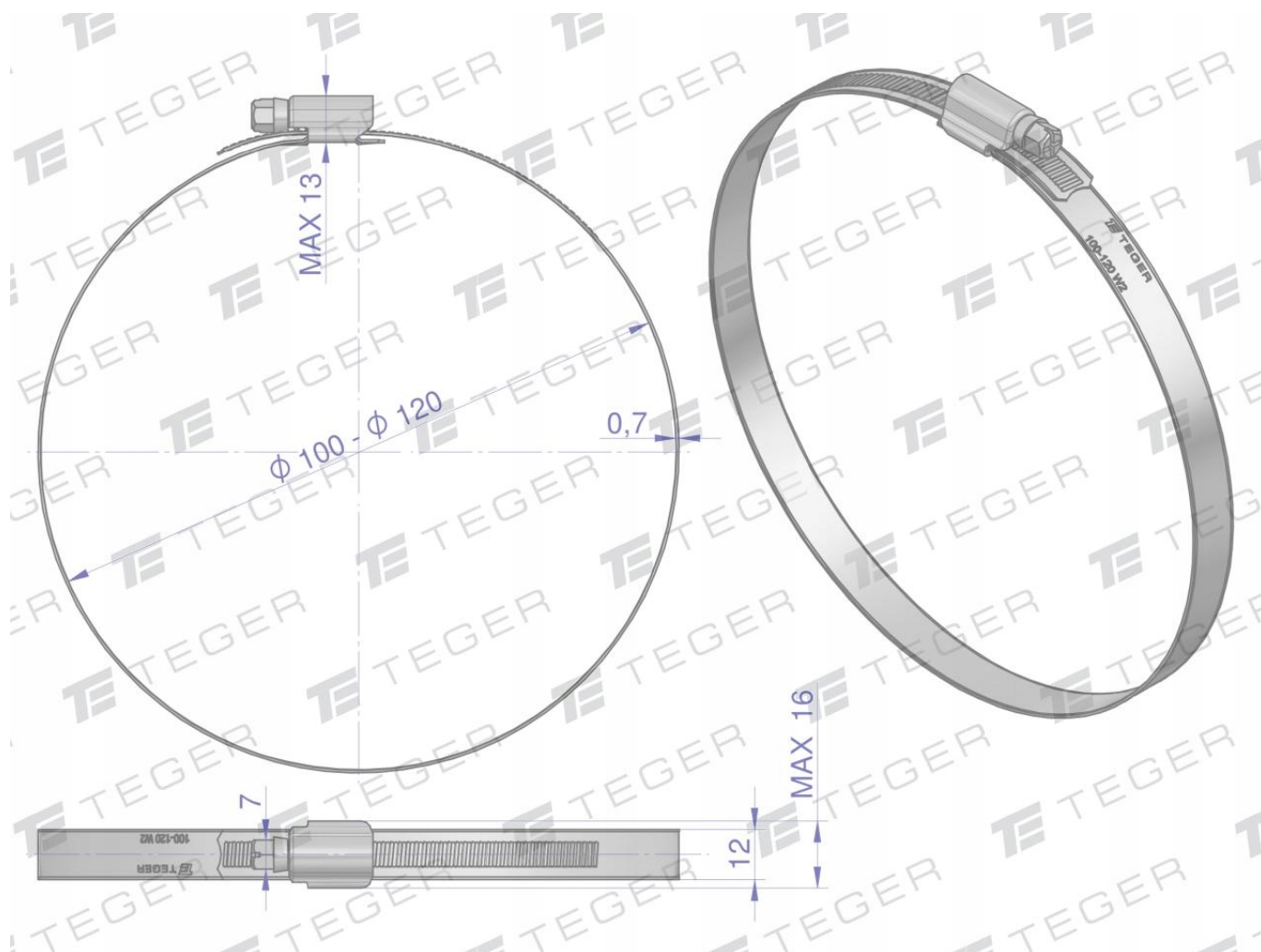
Opaska zaciskowa wzmacniana 100-120 ślimakowa skręcana (obejma W2 - stal nierdzewna) szerkość 12mm TEGER. Opaski zaciskowe ślimakowe - łatwe w montażu: śrubokręt lub klucz, trwałe, duża siła zaciskająca.
