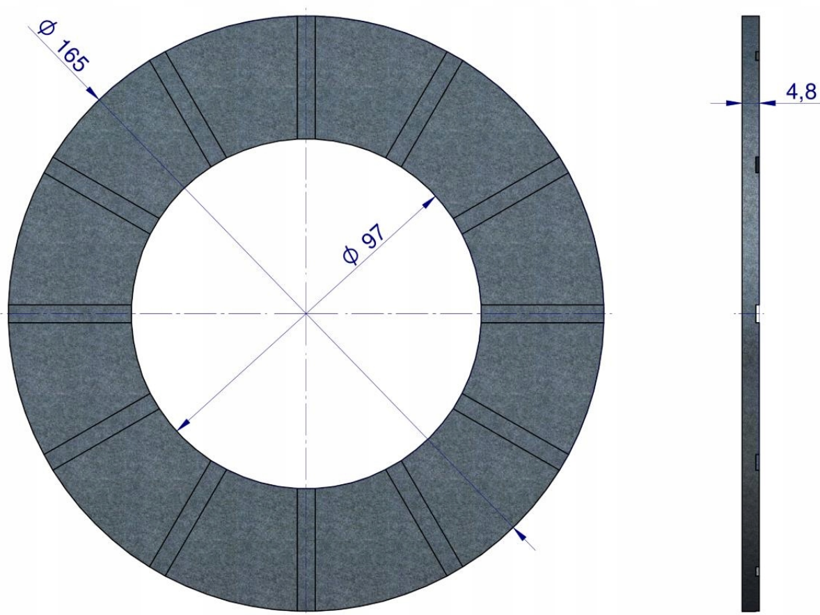
Okładzina sprzęgła ciernego wału przegubowo-teleskopowego seria 8 i 9 wymiary 165x97x4.8 WARYŃSKI
