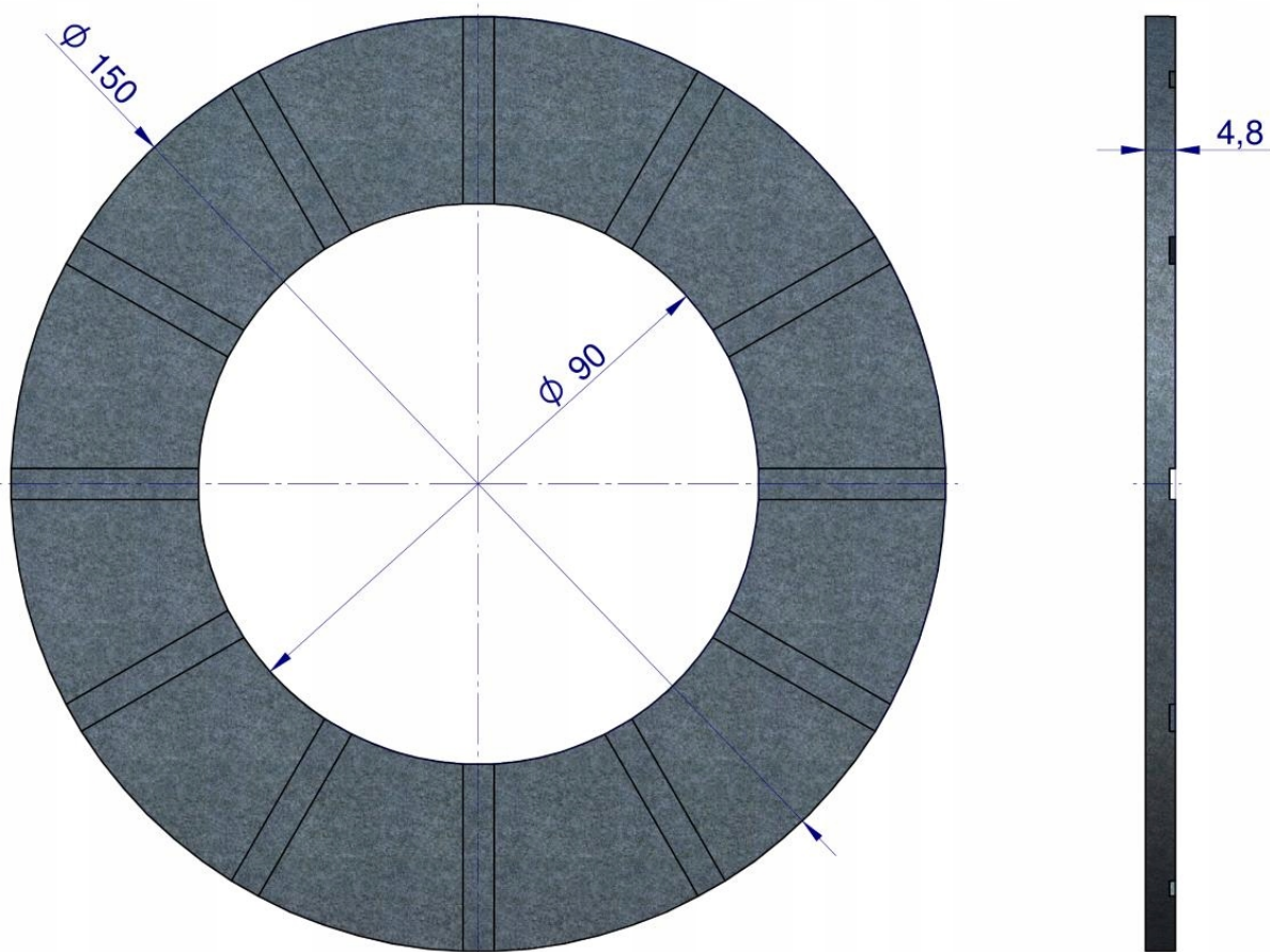
Okładzina sprzęgła ciernego wału przegubowo-teleskopowego seria 5 i 6 wymiary 150x90x4.8 WARYŃSKI
