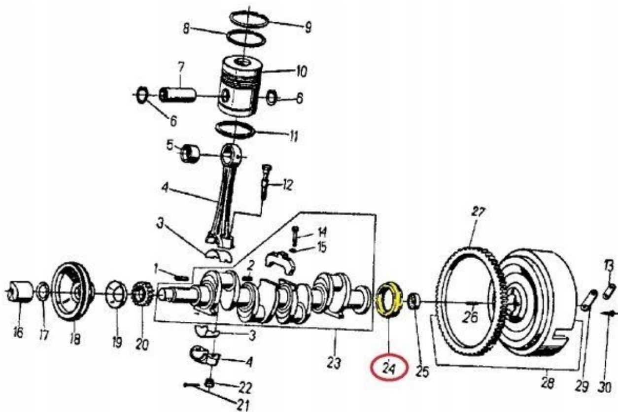
Odrzutnik tylny oleju Ursus C360
