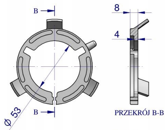
Pierścień wewnętrzny
