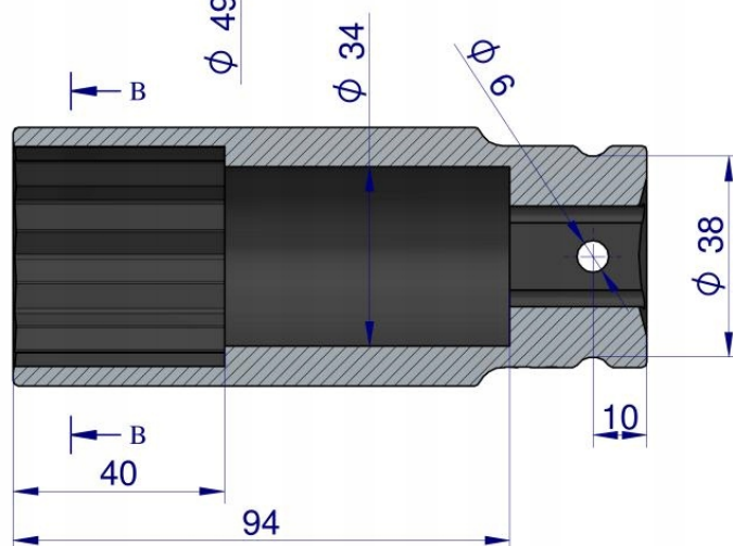
PRZEKRÓJ A-A
