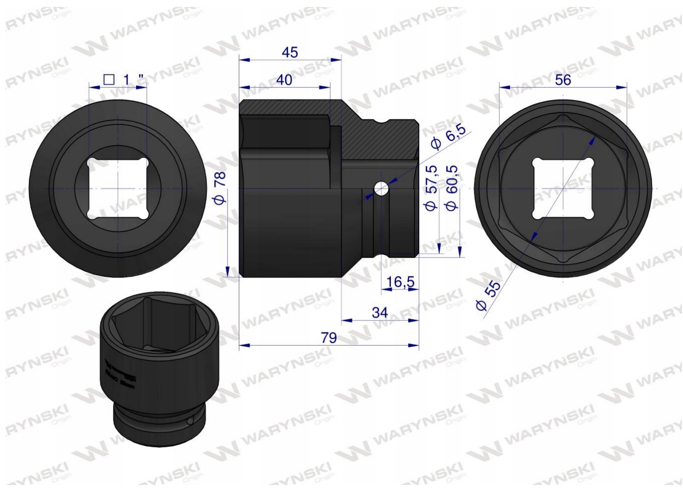
Nasadka udarowa 1 cal sześciokątna rozmiar 55mm z utwardzanej stali CrMo, przeznaczona do pracy z zastosowaniem uchwytu lub klucza udarowego Waryński
