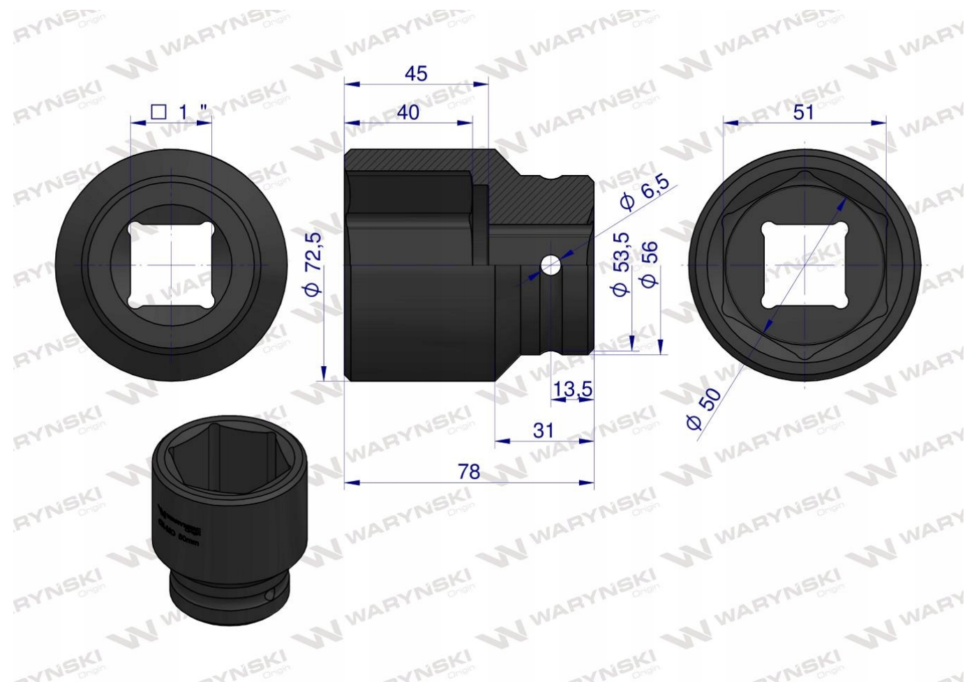
Nasadka uderowa 1 cal sześciokątna rozmiar 50mm z utwardzanej stali CrMo, przeznaczona do pracy z zastosowaniem uchwytu lub klucza uderowego Waryński
