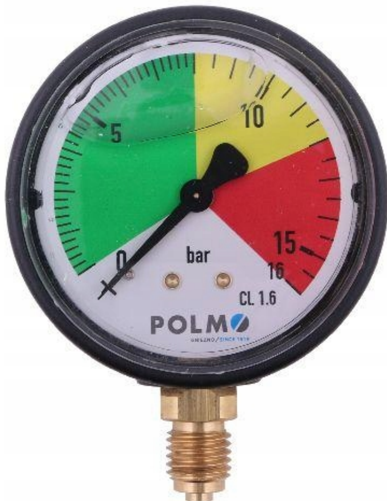
Manometr glicerynowy M63 0-16 bar, gwint M12x1,5 dolne przyłącze, obudowa plastikowa, Opryskiwacz POLMO
