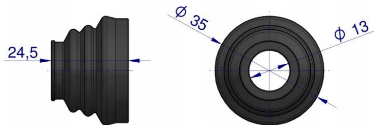
PRZEKRÓJ A-A
