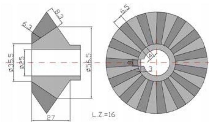
Koło zębate kosiarki małe Skropol Kosiarka rotacyjna
