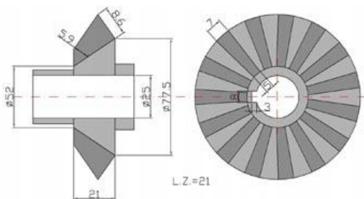
Koło zębate kosiarki duże Skropol Kosiarka rotacyjna
