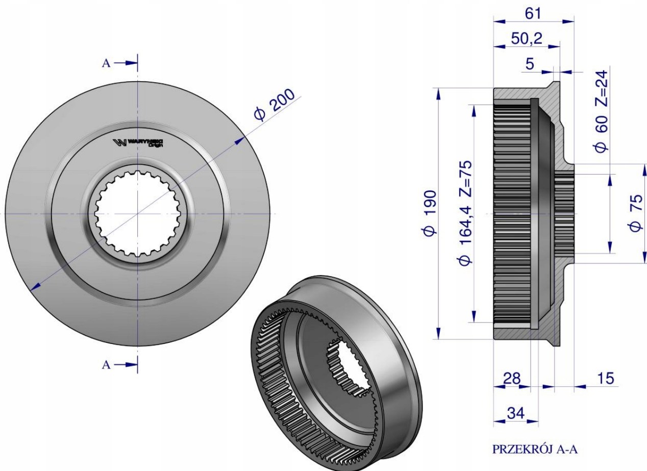
Koło koronowe C-385 80126107 WARYŃSKI
