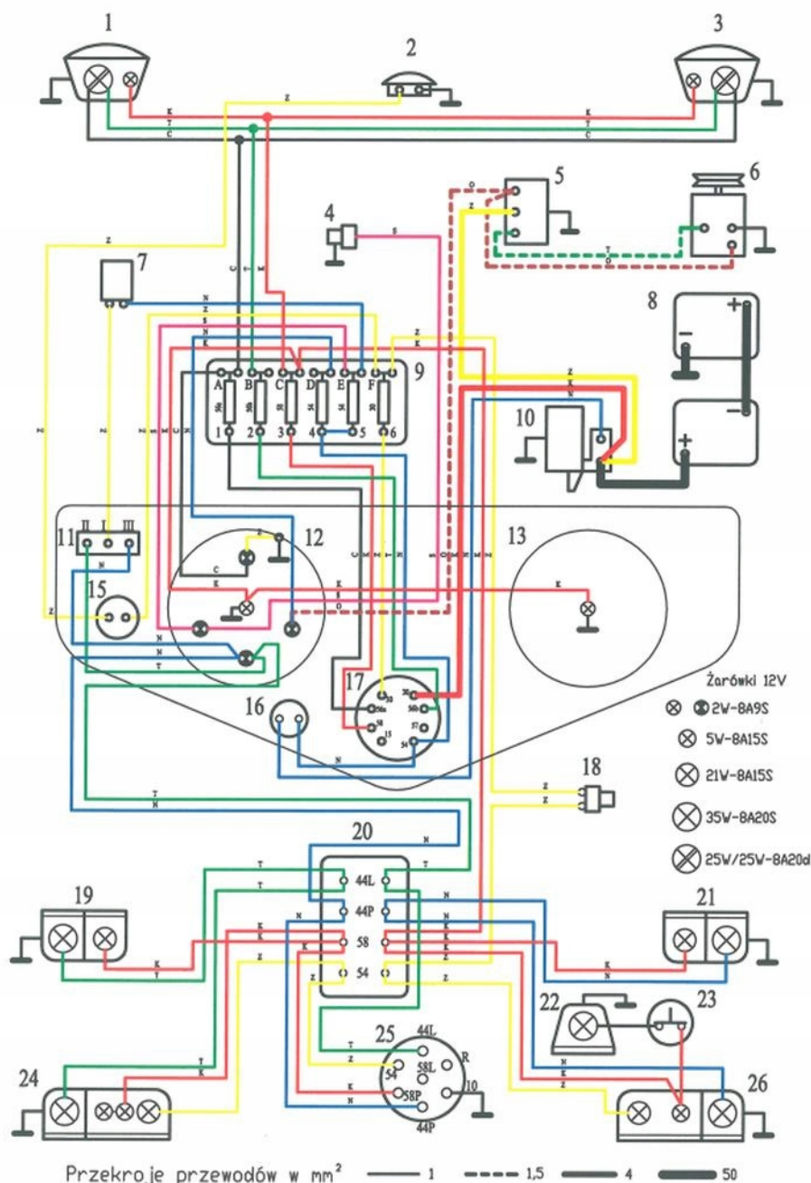
Schemat instalacji elektrycznej C-360 (prądnica)
