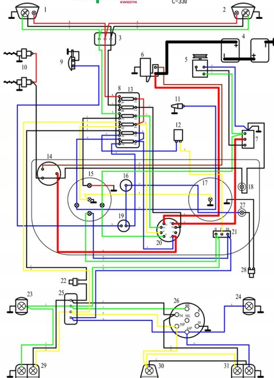
Schemat instalacji elektrycznej C-330 (prądnica)
