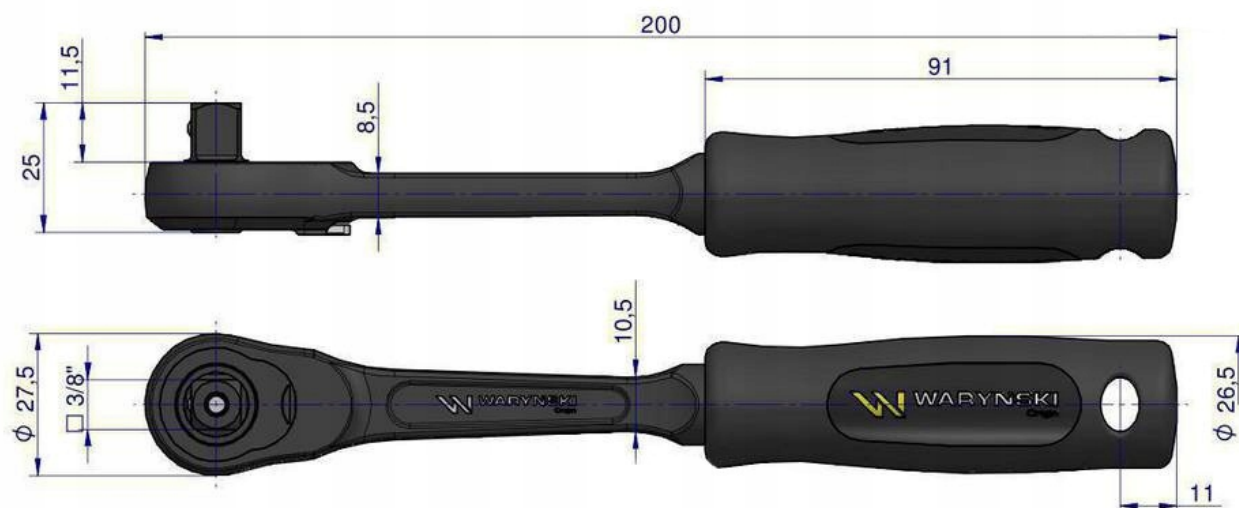
Mechanizm grzechotki
