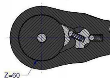
Mechanizm grzechotki
