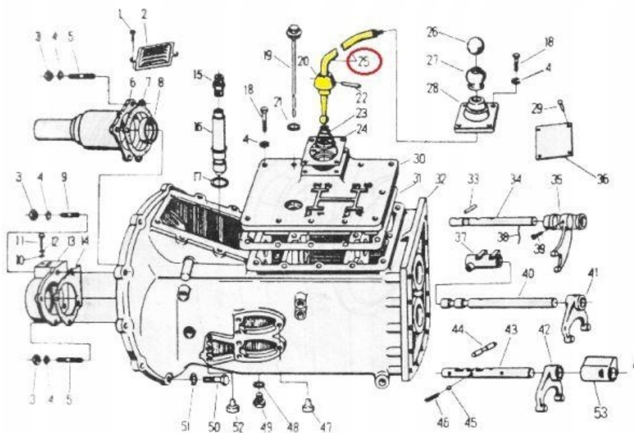
Dźwignia zmiany biegów C-330
