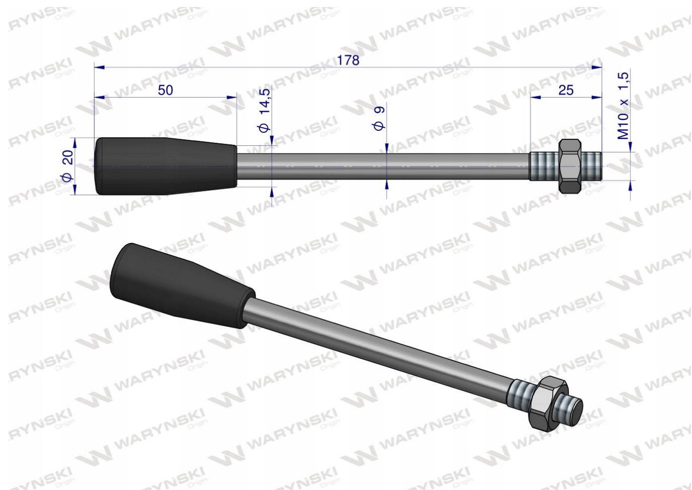
Dźwignia ręczna rozdzielacza
