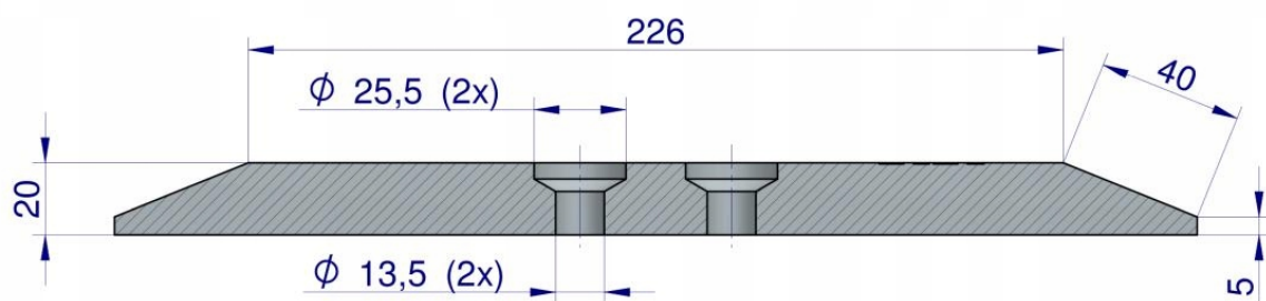
PRZEKRÓJ A-A
