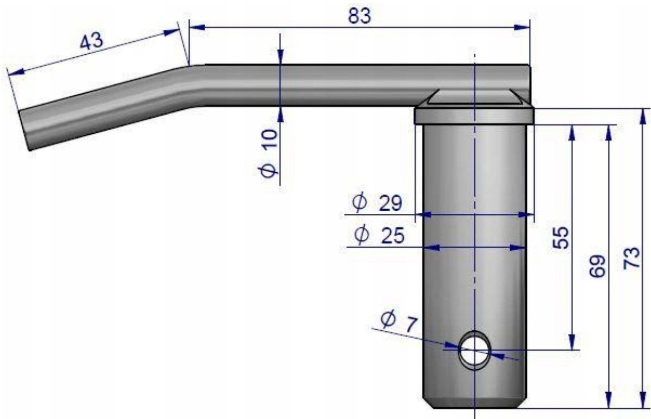
Czop (sworzeń) zabezpieczający mocowania nośnika zaczepu C385
